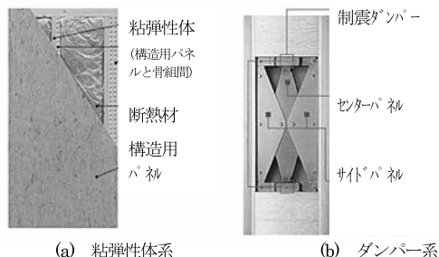
図2 戸建住宅用制震装置一例
